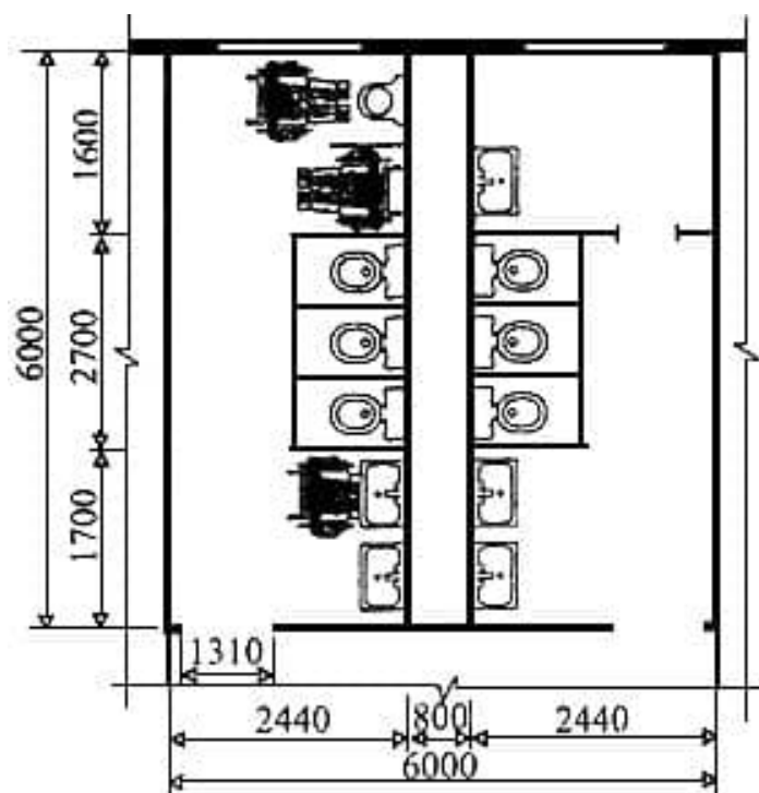
Цеховая уборная с кабиной для инвалидов
