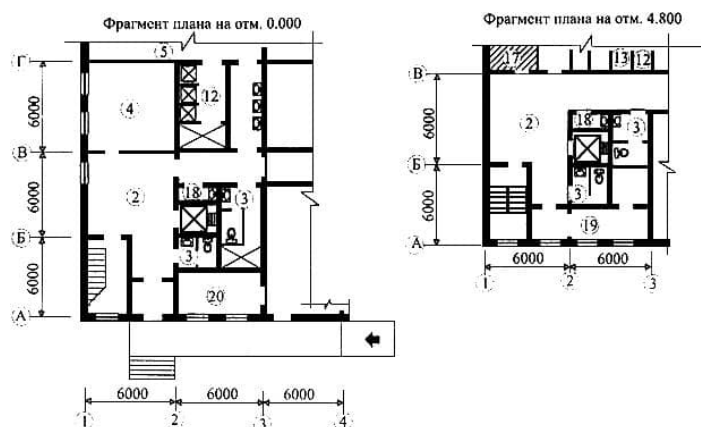
Рисунок В.14 - Адаптация цеха мучных изделий для обеспечения трудоустройства инвалидов
