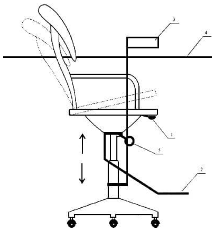
Рисунок В.12 - Трансформируемый рабочий стол для инвалида
