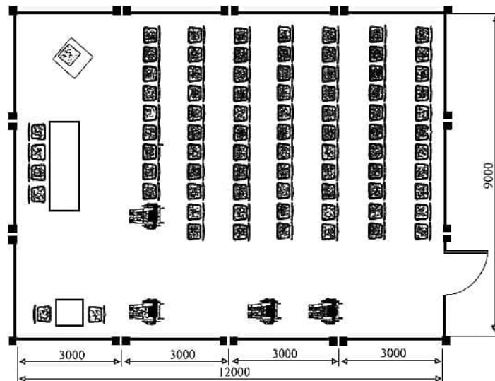
Рисунок В.5 - Помещения социального обслуживания
