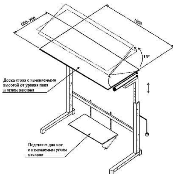
Рисунок В.12 - Трансформируемый рабочий стол для инвалида
