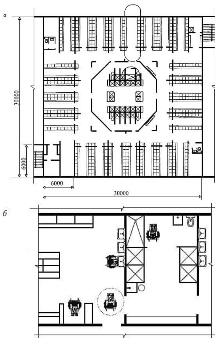
Размещение гардеробной (а) и душевой (б) для инвалидов в общем гардеробном блоке. Индивидуальная кабина инвалида в общей душевой
