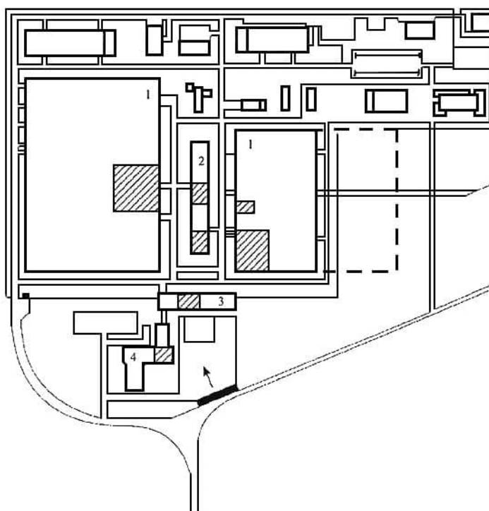
Рисунок В.2 - Встроенный контрольно-пропускной пункт
