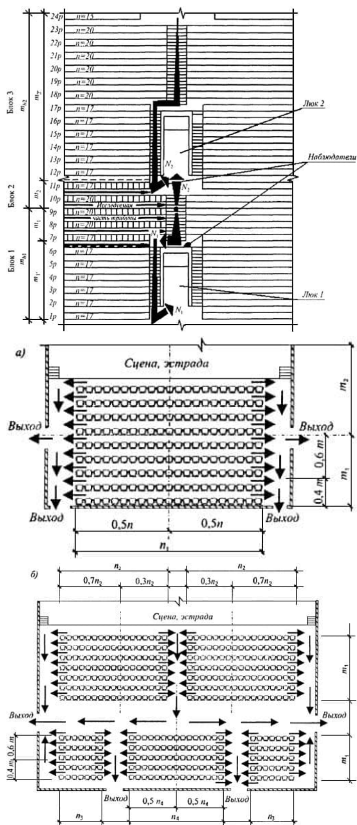
Рисунок И.1 - Маршрутизация движения людских потоков при эвакуации из зрительных залов
