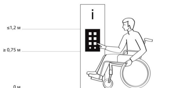
Рисунок 28 — Высота размещения рабочей зоны с элементами управления для информационных терминалов
