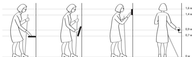
Рисунок 30 — Высоты размещения тактильной информации
