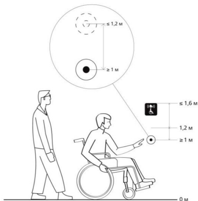
Рисунок 36 — Высота размещения кнопки
