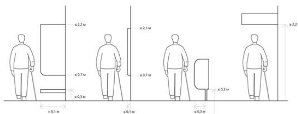
Рисунок В.2 — Выступы вдоль путей движения
