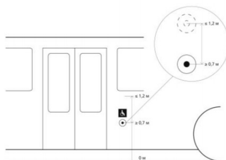
Рисунок 39 — Расположение кнопок персонала на поручнях транспортных средств вызова персонала на внешней стороне кузова транспортных средств
