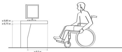
Рисунок Б.6 — Высота рабочей поверхности для обслуживания инвалида, использующего для передвижения кресло-коляску
