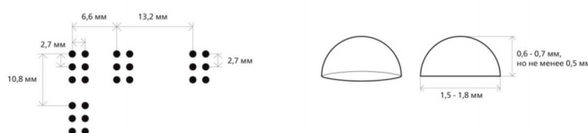
Рисунок 31 — Размеры рельефно-точечного шрифта Брайля
