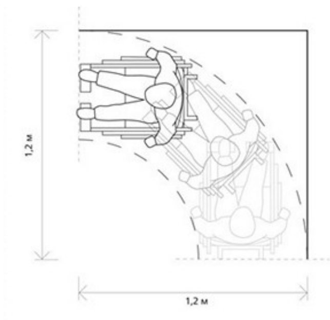
Рисунок Б.2 — Пространство для поворота на 90^\circ
