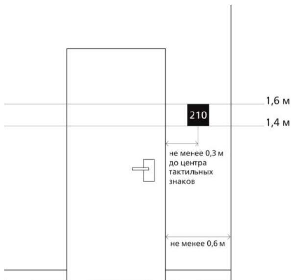
Рисунок 9 — Размещение информации относительно полотна двери
