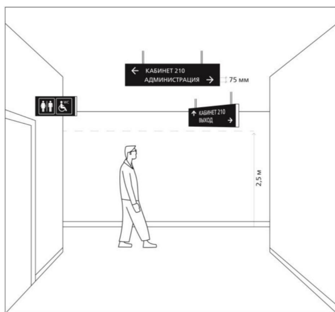
Рисунок 3 — Размер знаков на технических визуальных средствах информации, размещенных на высоте более 2,5 м, и принцип размещения в интерьере указателей, расположенных на консолях и на подвесных кронштейнах
