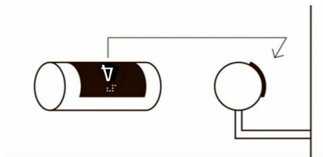
Рисунок 35 — Размещение тактильной информации на поручнях (вид таблички со стороны стены)
