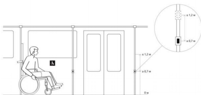
Рисунок 38 — Расположение кнопок вызова
