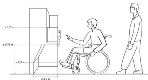
Рисунок Б.5 — Размеры глубины и высоты проема для ног при фронтальном подходе к оборудованию
