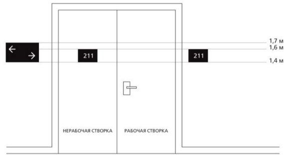
Рисунок 8 — Вариант размещения информации на нерабочих створках дверей
