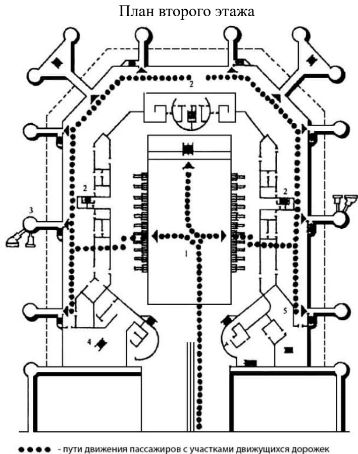
1 - операционный зал; 2 - зал вылета; 3 - посадочные сооружения; 4 - сектор для отдыха физически ослабленных лиц, инвалидов; 5 - сектор "Интурист" Рисунок В.10 - Организация движения пассажиров в аэровокзале
