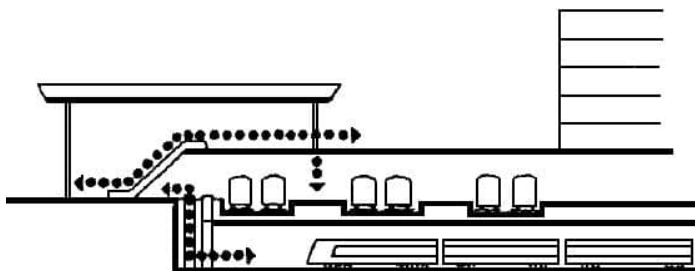
Рисунок В.5 - Приемы организации движения пассажиров в вокзальных комплексах различного назначения*
